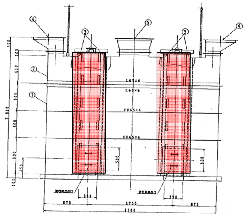
A-A侧面图
