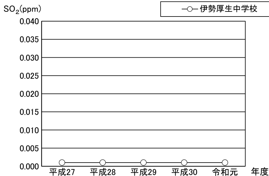
図 3-4 二酸化硫黄年平均値の経年変化（平成27年度～令和元年度）
