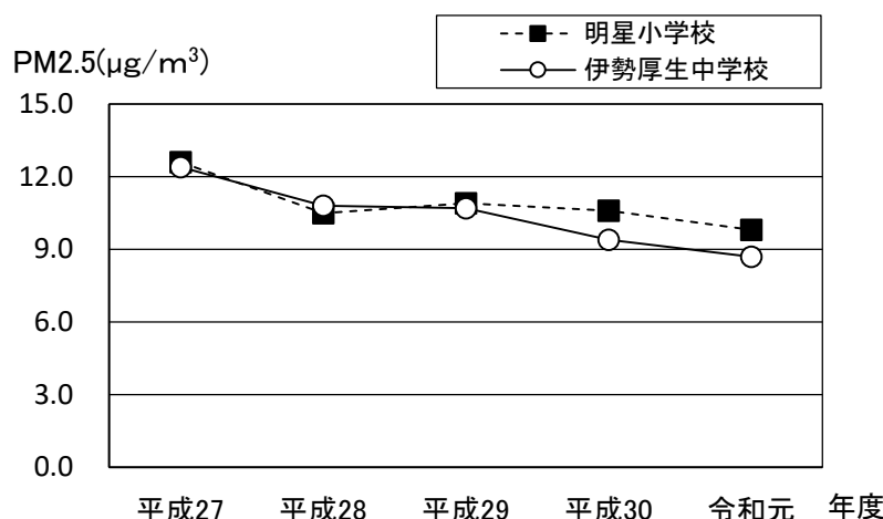
図 3-7 微小粒子状物質年平均値の経年変化 (平成27年度～令和元年度)
