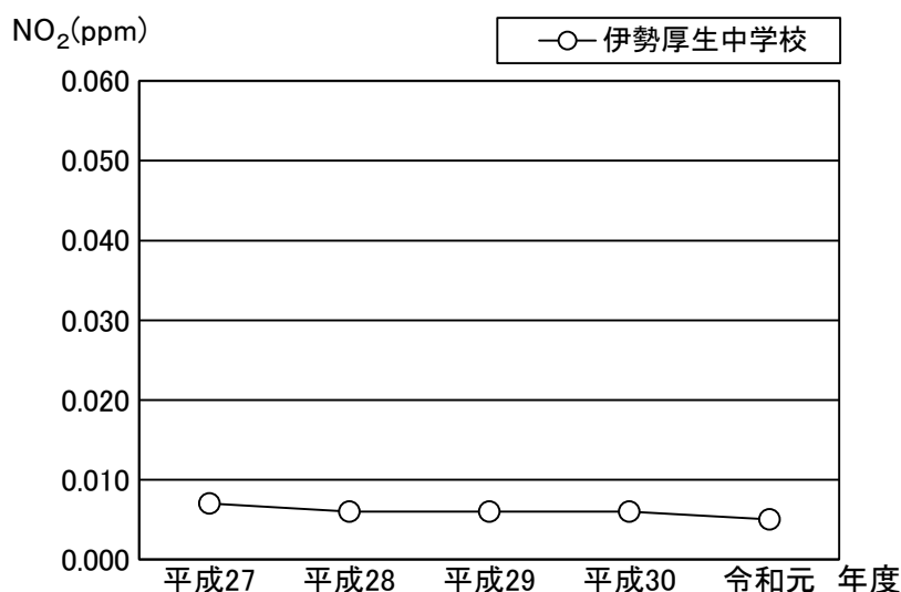
図 3-5 二酸化窒素年平均値の経年変化（平成27年度～令和元年度）
