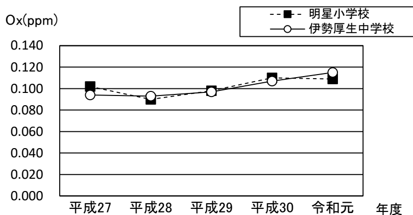
図 3-8 光化学オキシダント(昼間の1時間値の最高値)の経年変化(平成27年度～令和元年度)
