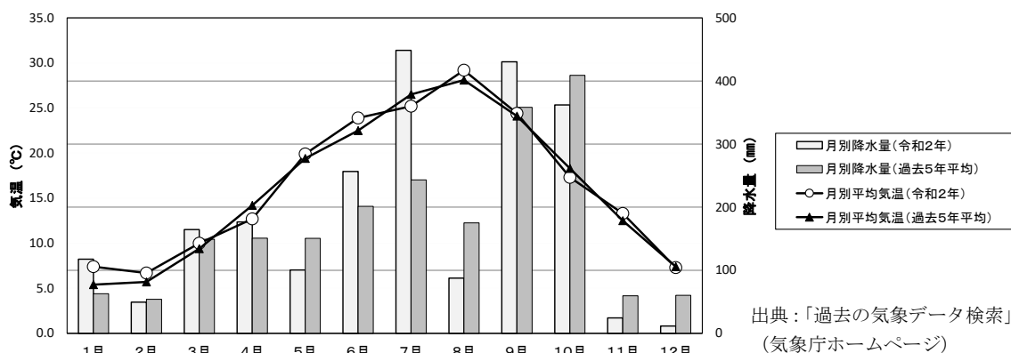
図 3-2 小俣気象観測所における月別平均気温及び降水量（平成28年～令和2年）
