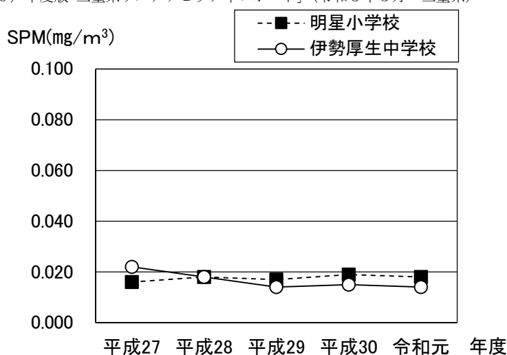
図 3-6 浮遊粒子状物質年平均値の経年変化 (平成27年度～令和元年度)
