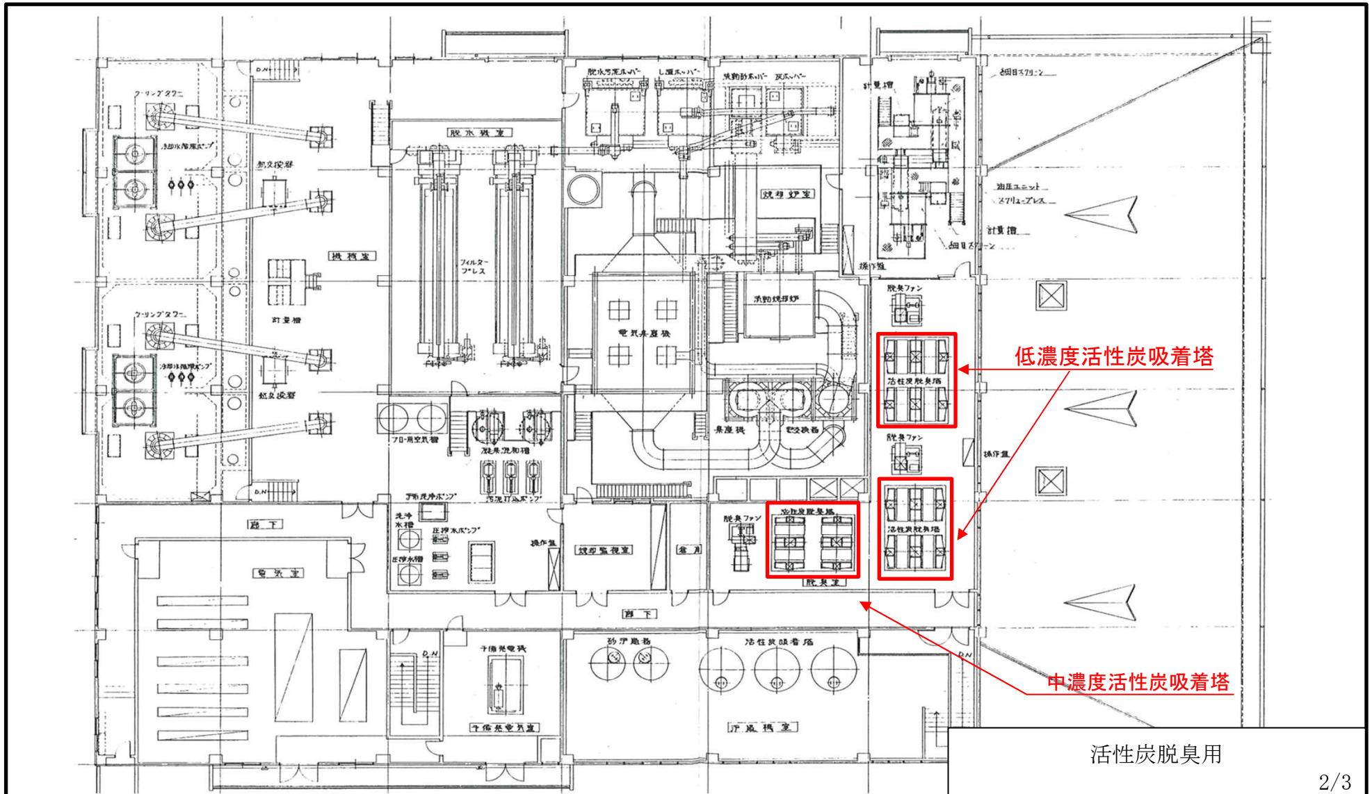
機器配置図 (2F)
